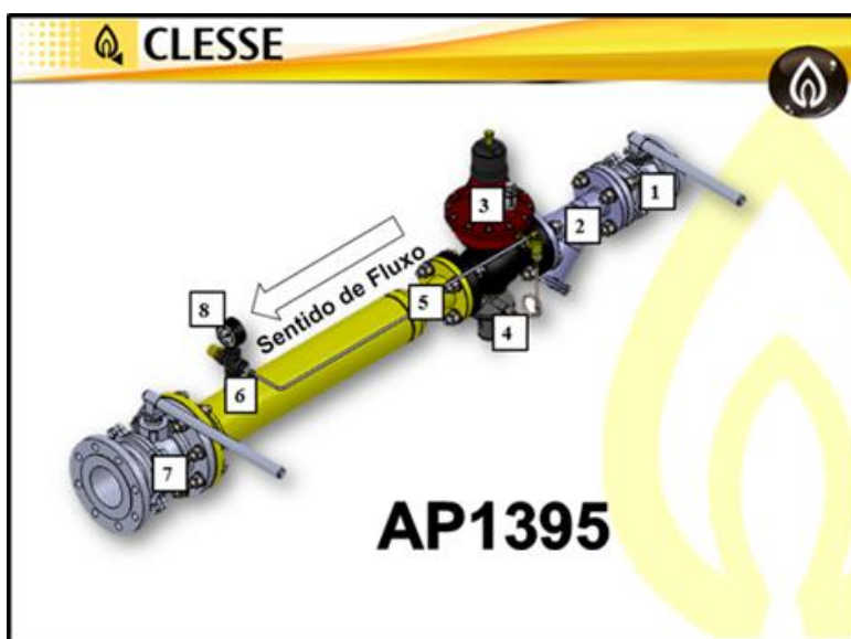
Figura 1 – instalação da tomada de impulso
